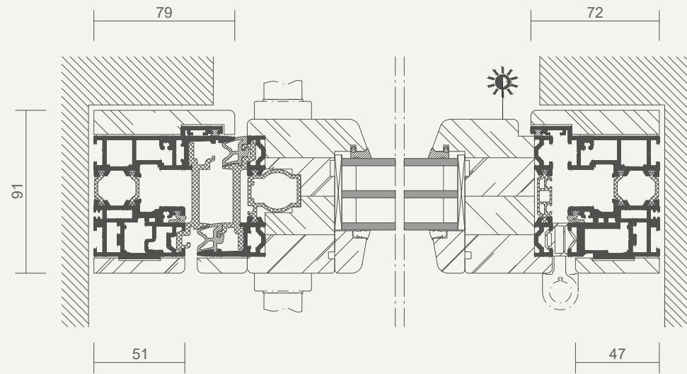
Horizontalschnitt
