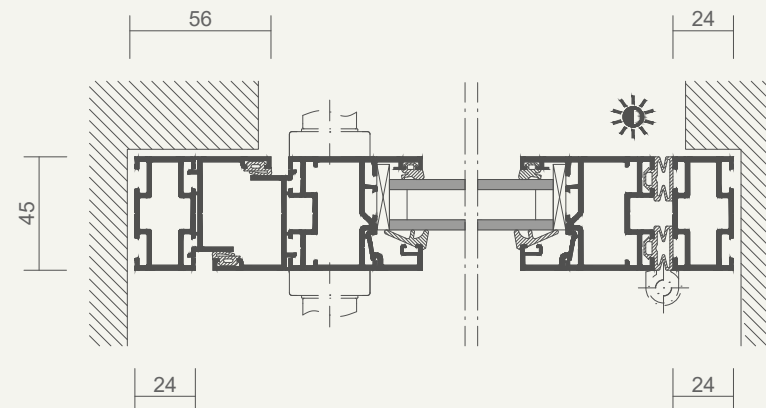
Horizontalschnitt
