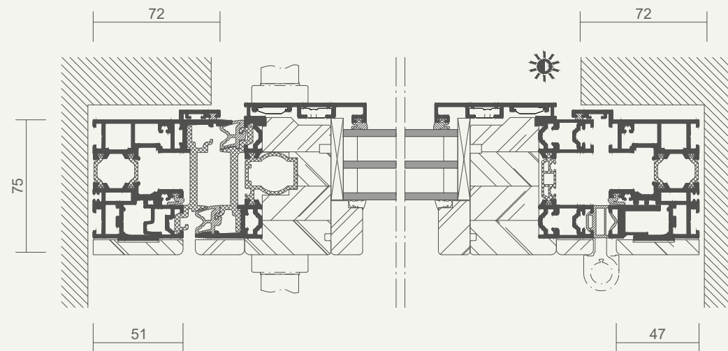
Horizontalschnitt
