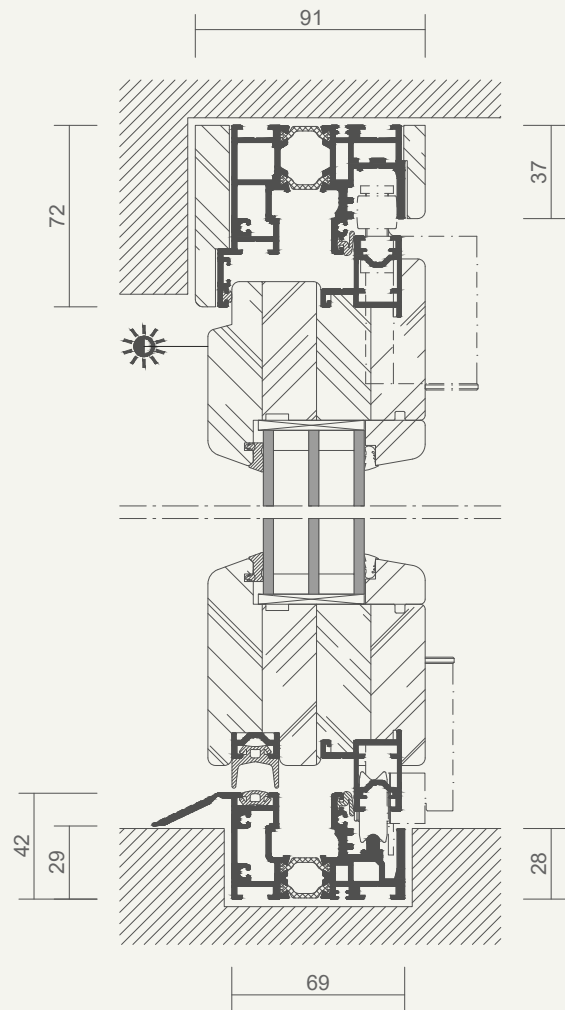
Vertikalschnitt
